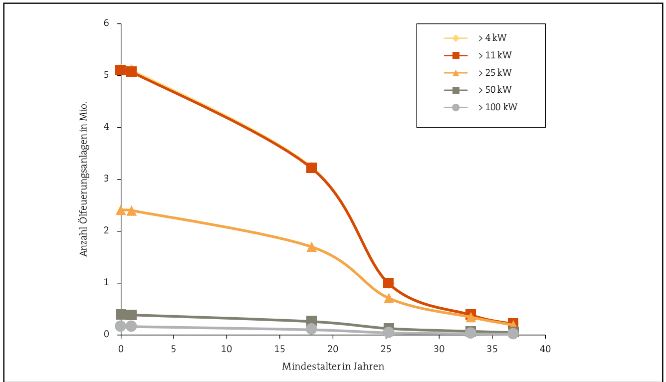
Altersstruktur der nach 1. BImSchV messpflichtigen Ölfeuerungsanlagen in Deutschland 2015 (ohne Brennwertfeuerstätten)
